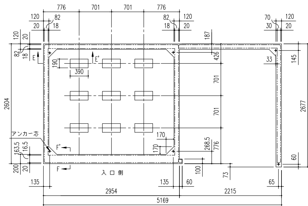
布基礎伏図 (S=1/50)
