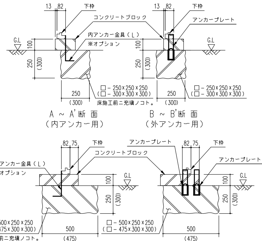
ブロック基礎断面図例 (S=1/20)
