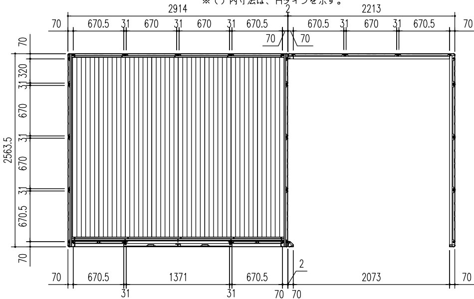
平面図 (S = 1/50)
