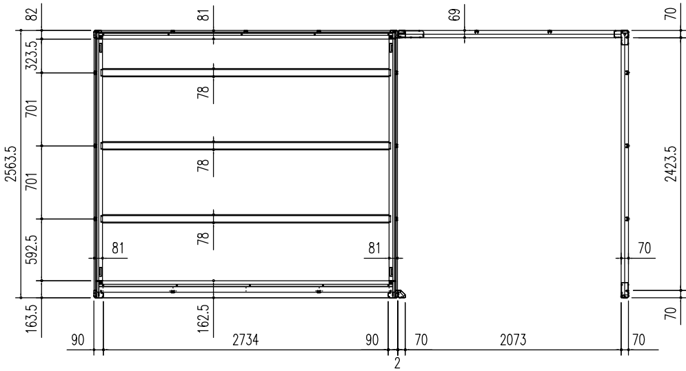
床伏図 (S = 1/50)
