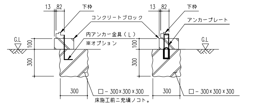
A ~ A' 断面 (内アンカー用)
