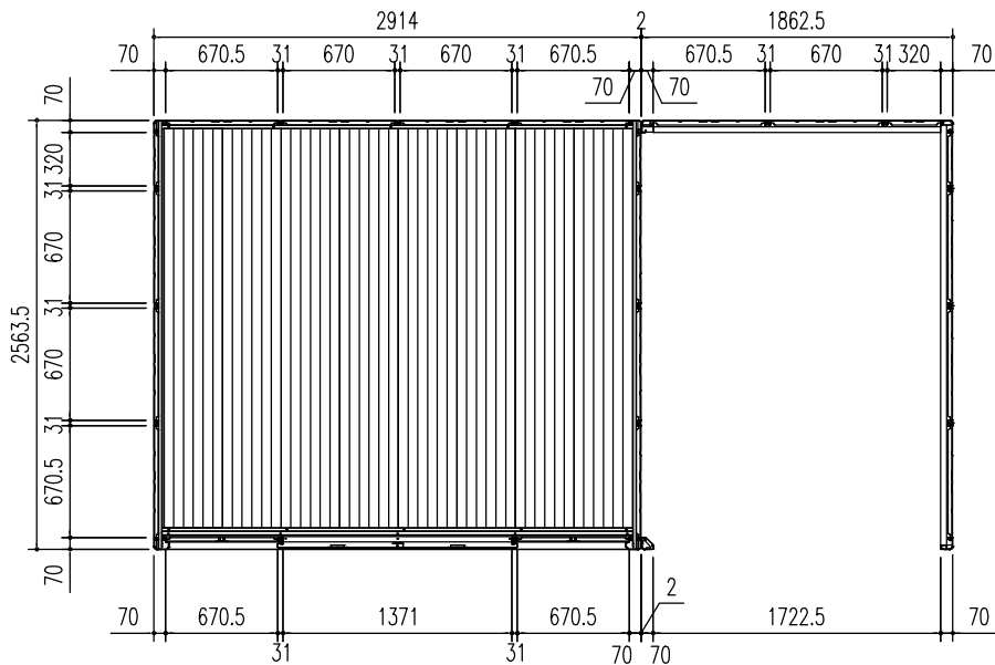
平面図 (S=1/50)
