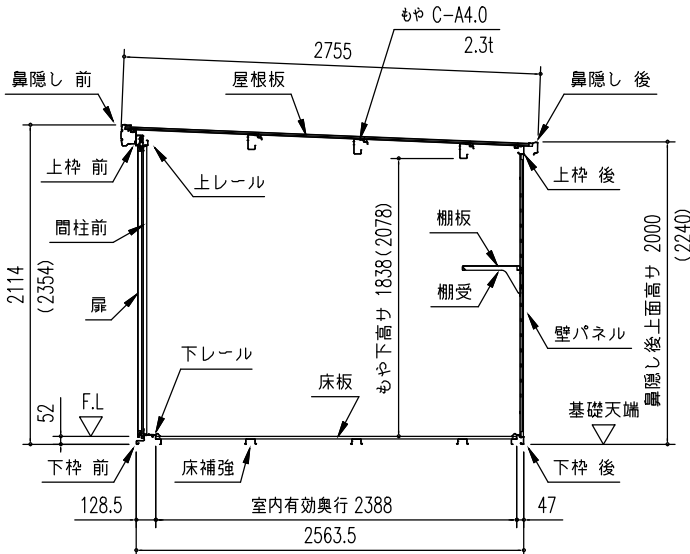
〔物置部〕矩計図 (S=1/50)
