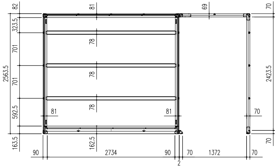
床伏図 (S=1/50)
