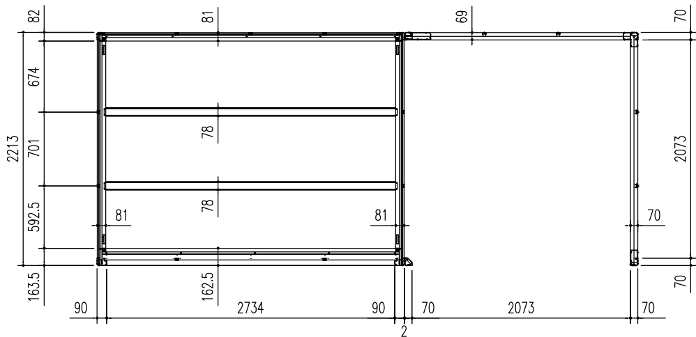
床伏図 (S = 1/50)
