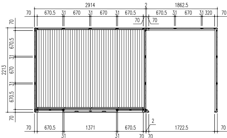
平面図 (S=1/50)
