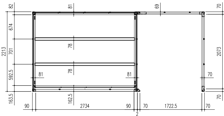
床伏図 (S=1/50)
