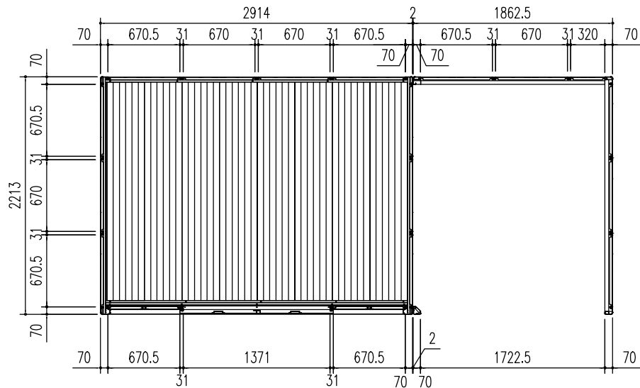
平面図 (S=1/50)
