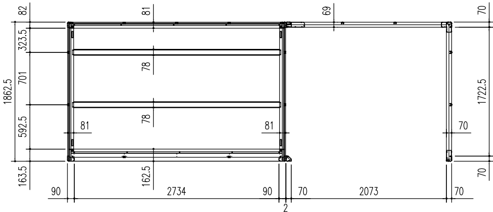
床 伏 図 (S = 1/50)
