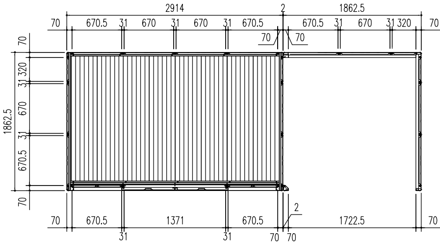
平面図 (S = 1/50)
