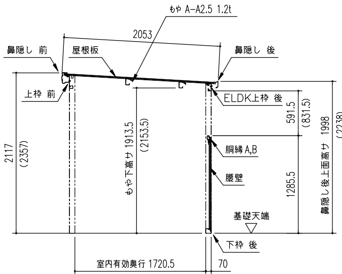
〔オープン部〕矩計図 (S = 1/50) ※ ( ) 内寸法は、Hタイプを示す。
