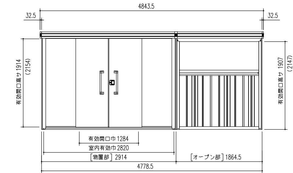
正面立面図 (S = 1/50) ※ ( ) 内寸法は、Hタイプを示す。
