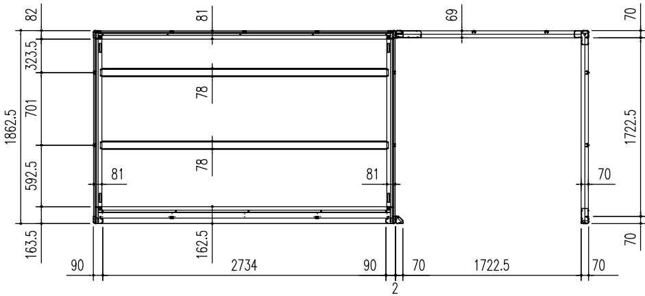
床伏図 (S = 1/50)
