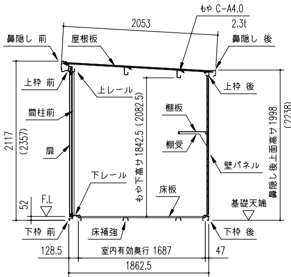
〔物置部〕矩計図 (S = 1/50) ※ ( ) 内寸法は、Hタイプを示す。
