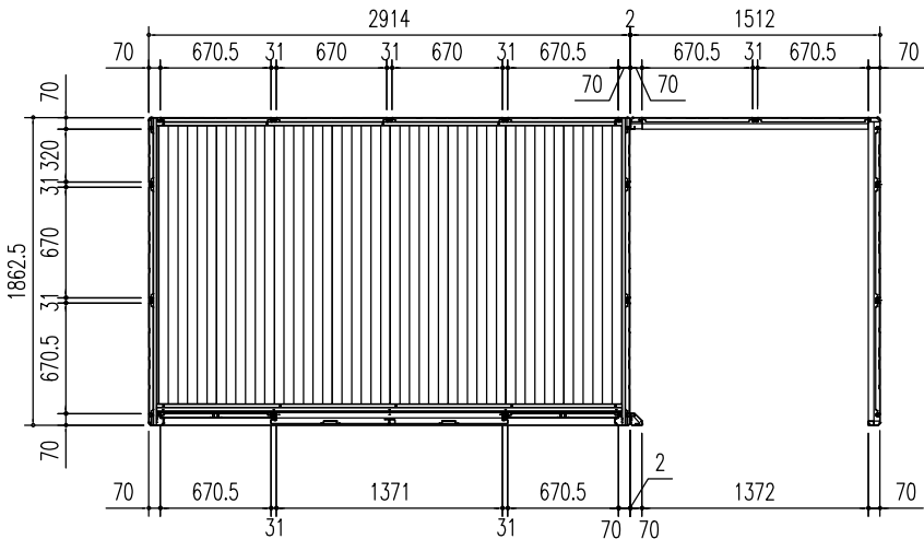
平面図 (S=1/50)
