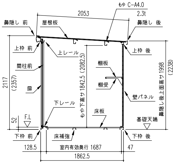
側面立面図 (S=1/50) ※( ) 内寸法は、Hタイプを示す。
