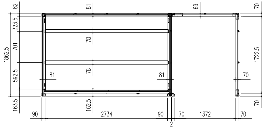
床伏図 (S = 1/50)
