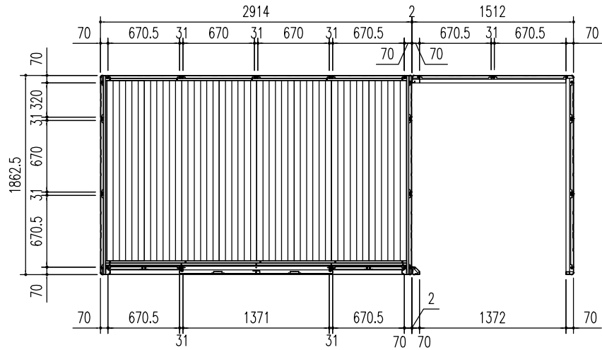
平面図 (S = 1/50)
