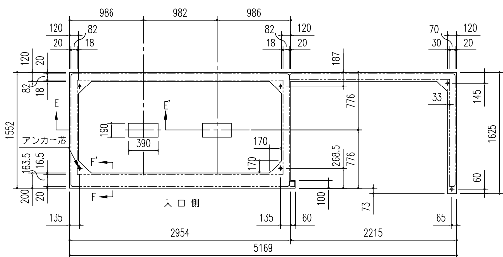
布基礎伏図 (S=1/50)
