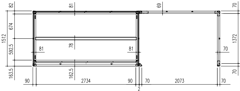
床伏図 (S=1/50)
