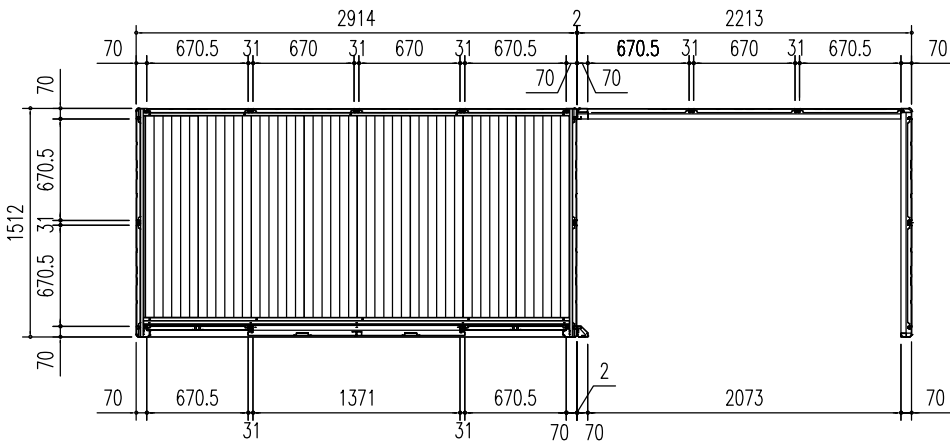
平面図 (S=1/50)
