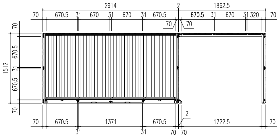
平面図 (S=1/50)
