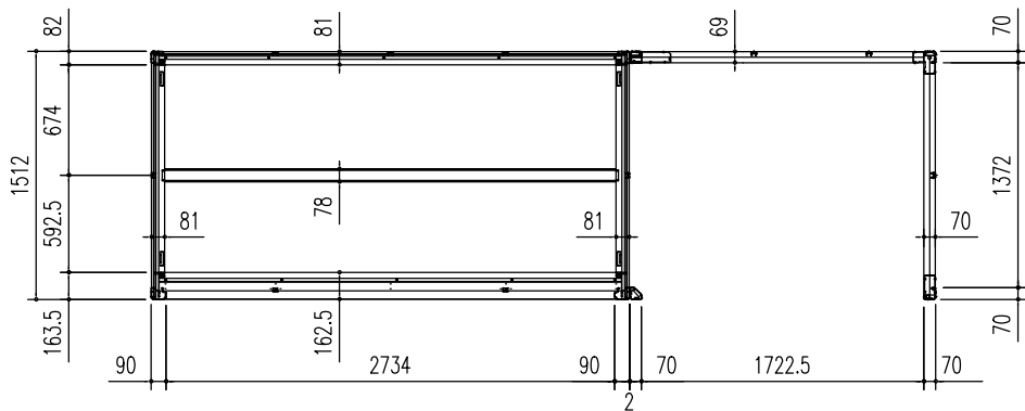
床伏図 (S=1/50)
