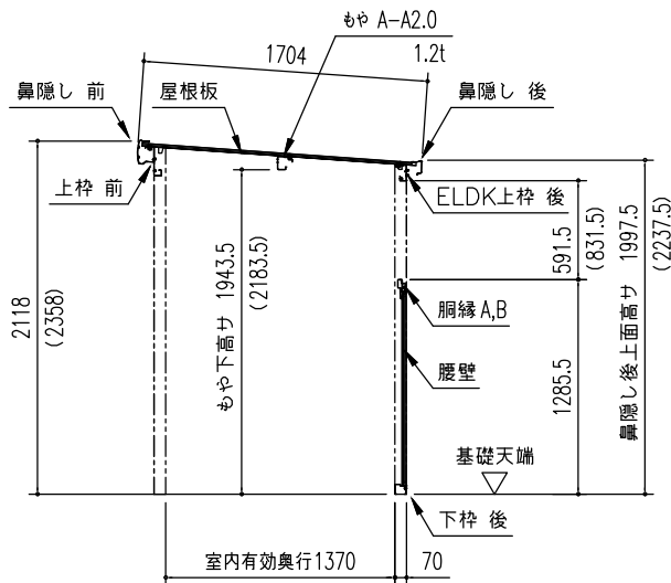
〔オープン部〕矩計図 (S=1/50)
