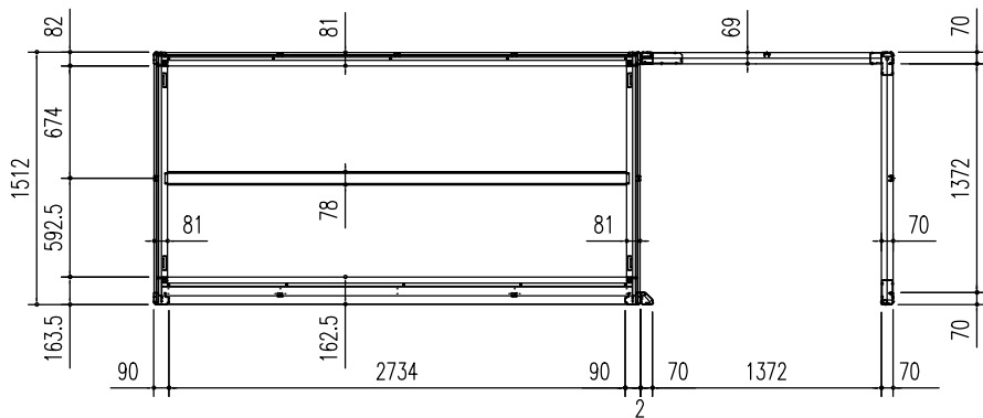
床伏図 (S=1/50)
