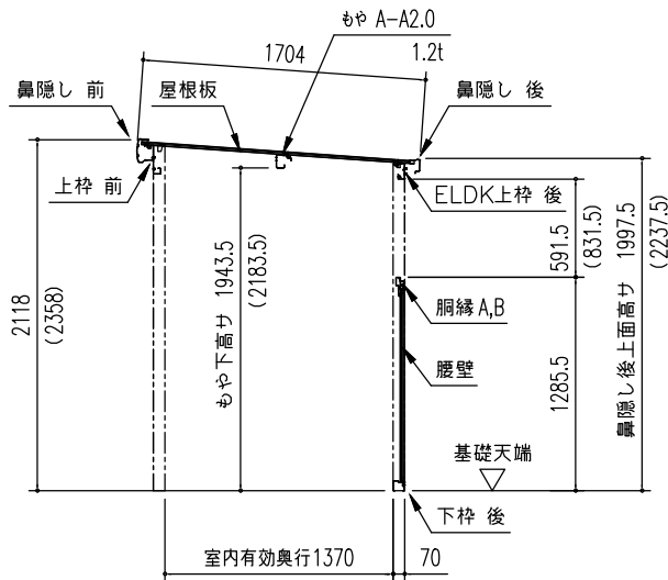
〔オープン部〕矩計図 (S = 1/50) ※ ( ) 内寸法は、Hタイプを示す。
