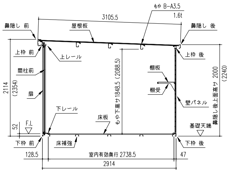
〔物置部〕矩計図
