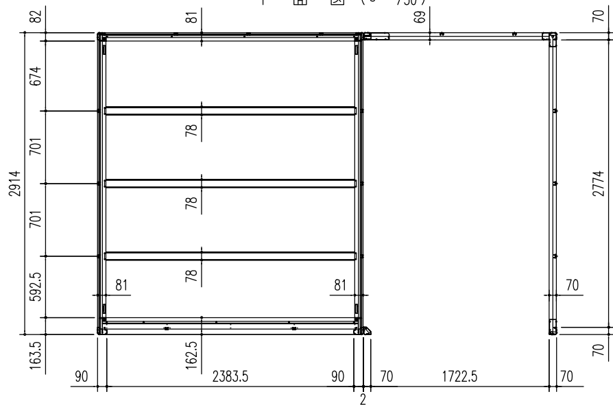
床 伏 図 (S = 1/50)
