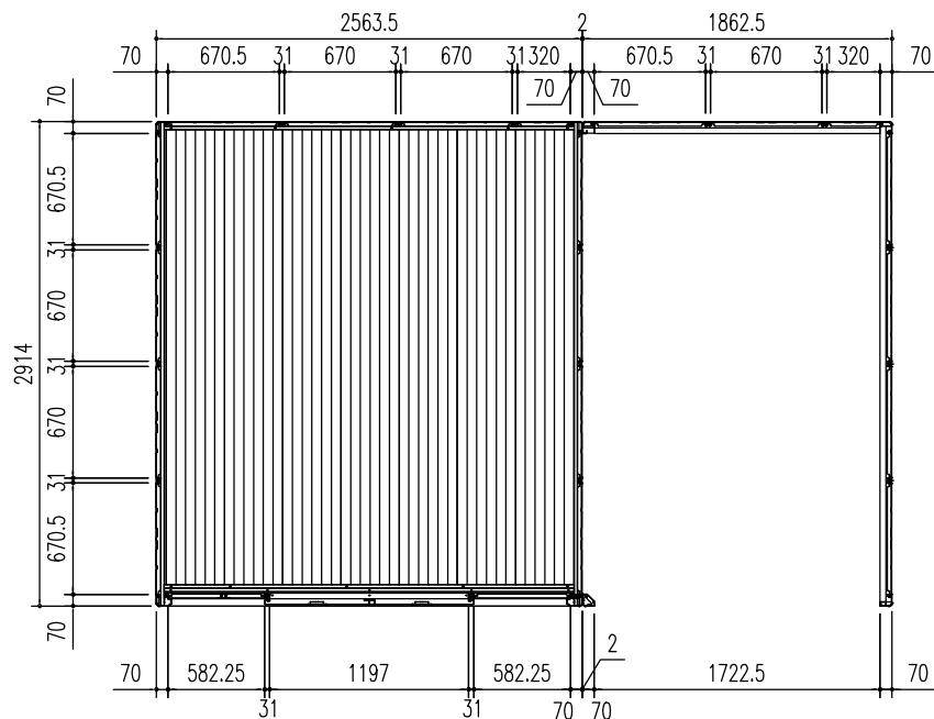
平面図 (S = 1/50)
