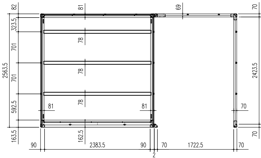
床伏図 (S = 1/50)
