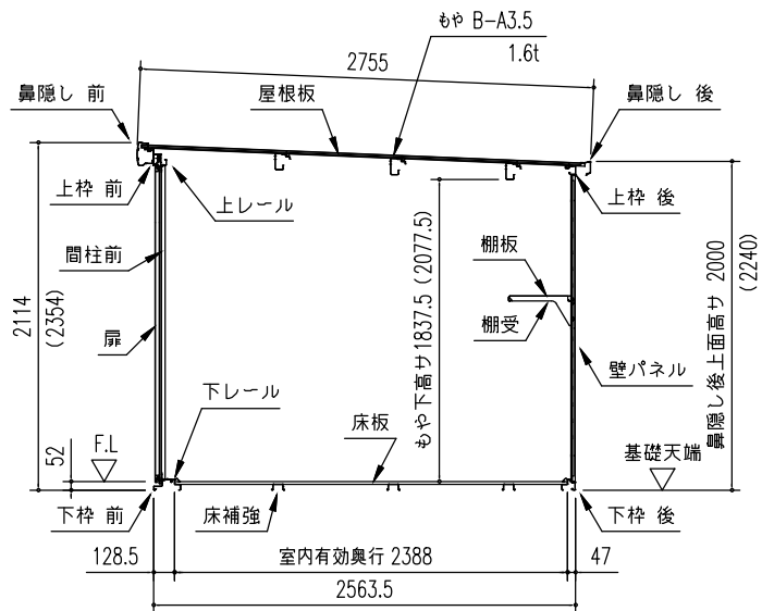
〔物置部〕矩計図
