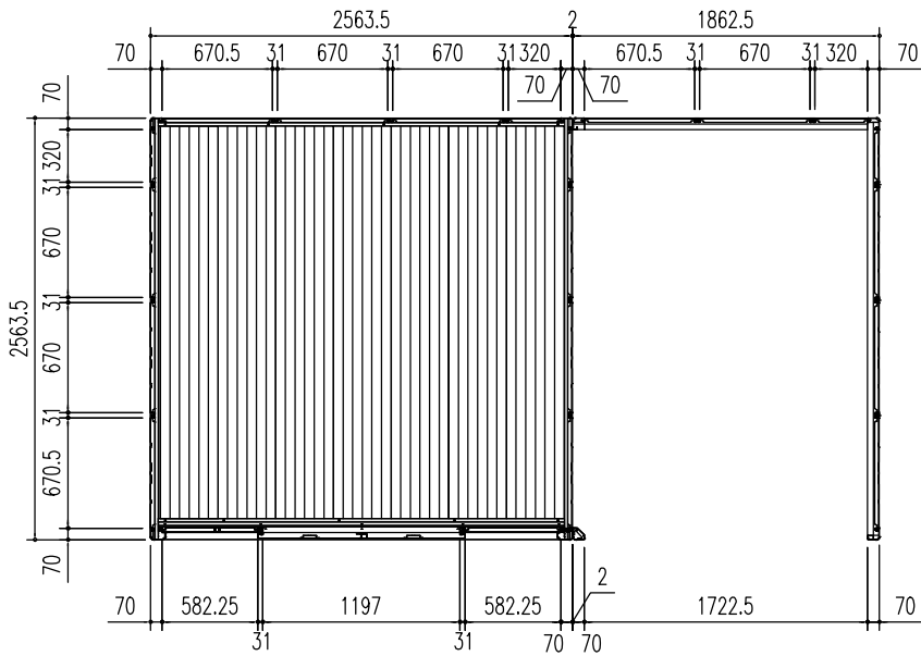
平面図 (S = 1/50)
