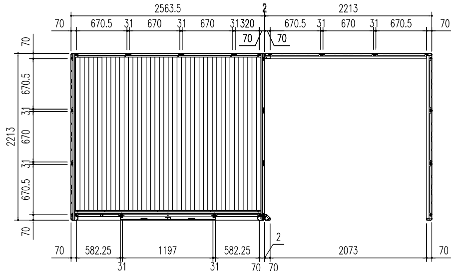
平面図 (s = 1/50)
