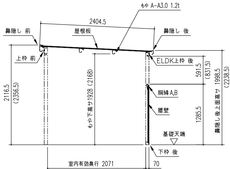
矩計図 (s = 1/50)
