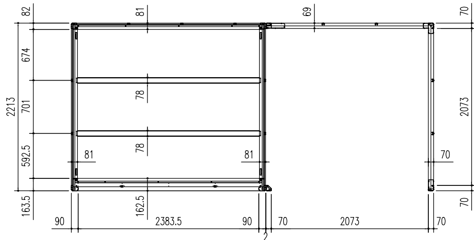
床伏図 (s = 1/50)
