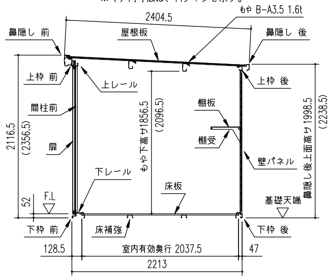
矩計図 (s = 1/50)
