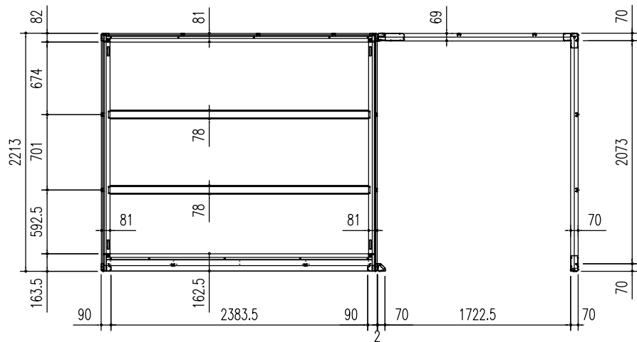
床伏図 (S = 1/50)
