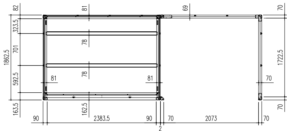
床伏図 (S = 1/50)
