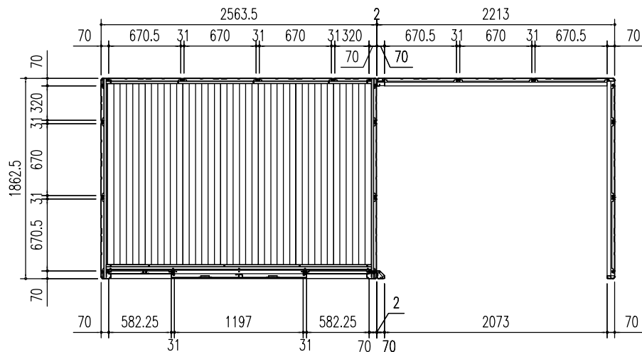
平面図 (S = 1/50)
