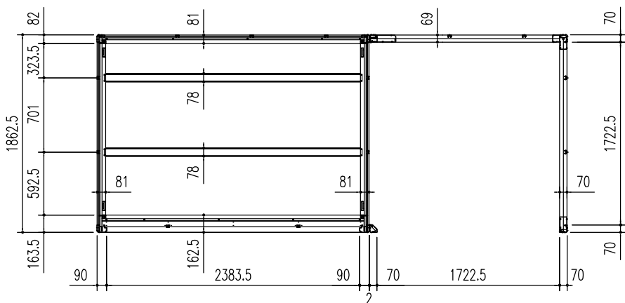
床伏図 (S = 1/50)
