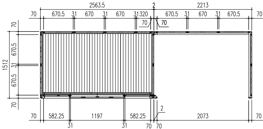
平面図 (S=1/50)
