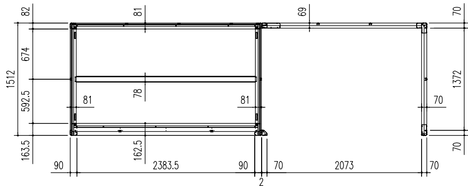
床伏図 (S=1/50)
