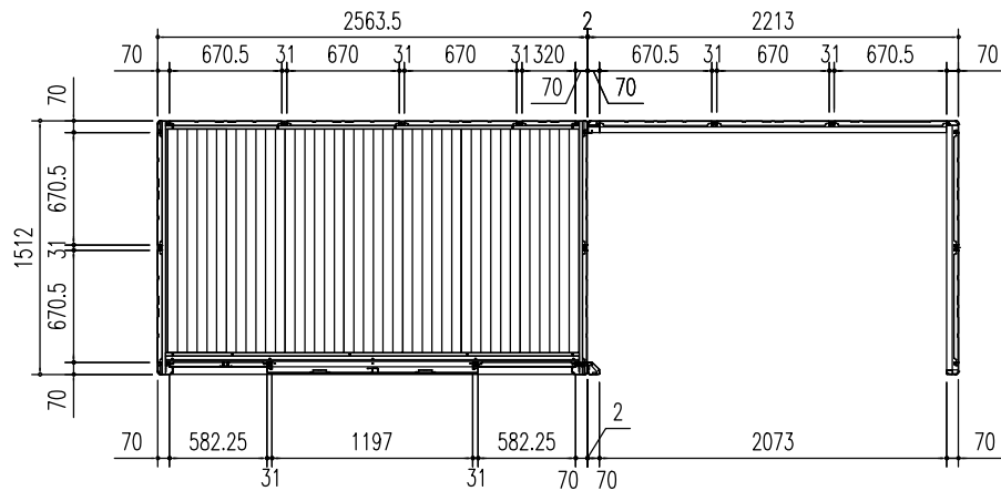
平面図 (S=1/50)
