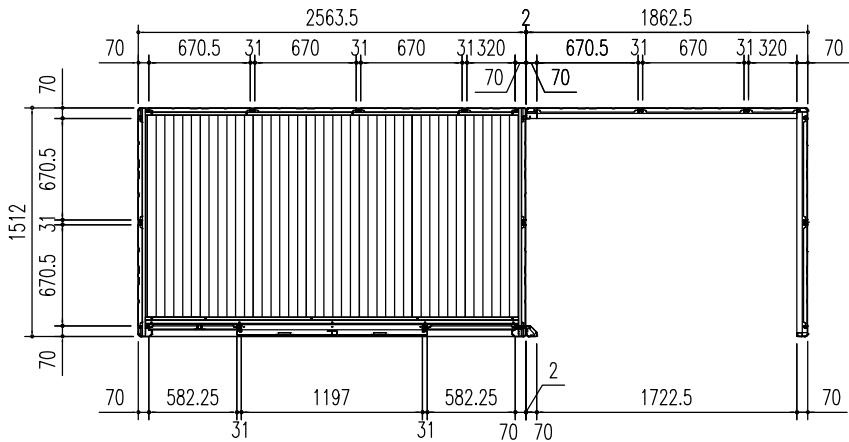
平面図 (S=1/50)
