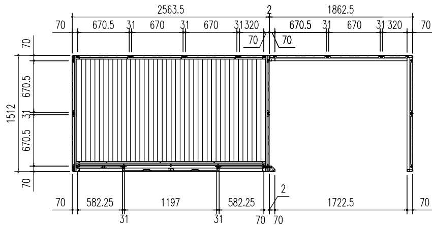
平面図 (S=1/50)
