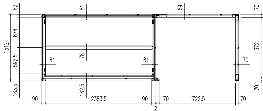
床伏図 (S=1/50)
