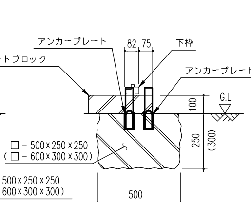
D ~ D' 断面 (外アンカー用)
