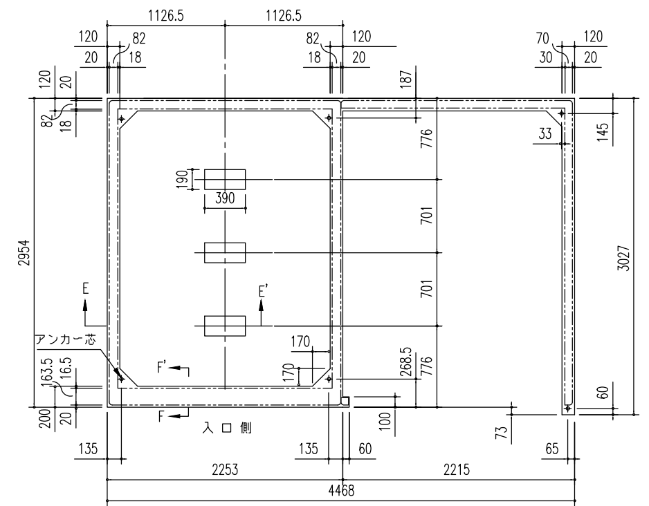
布基礎伏図 (S=1/50)
