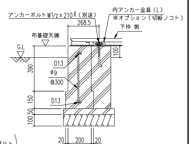
F ~ F' 断面
