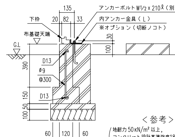
E ~ E' 断面
