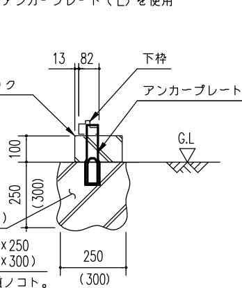
B ~ B' 断面 (外アンカー用)
