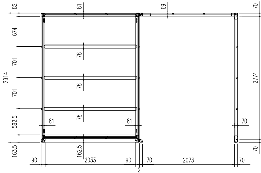
床伏図 (S=1/50)
