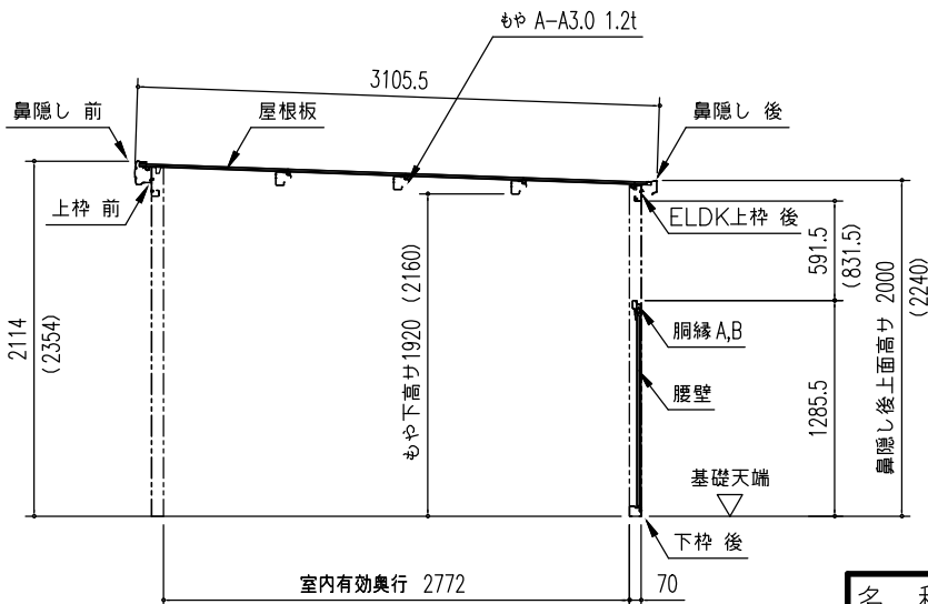
〔オープン部〕矩計図 (S=1/50)
