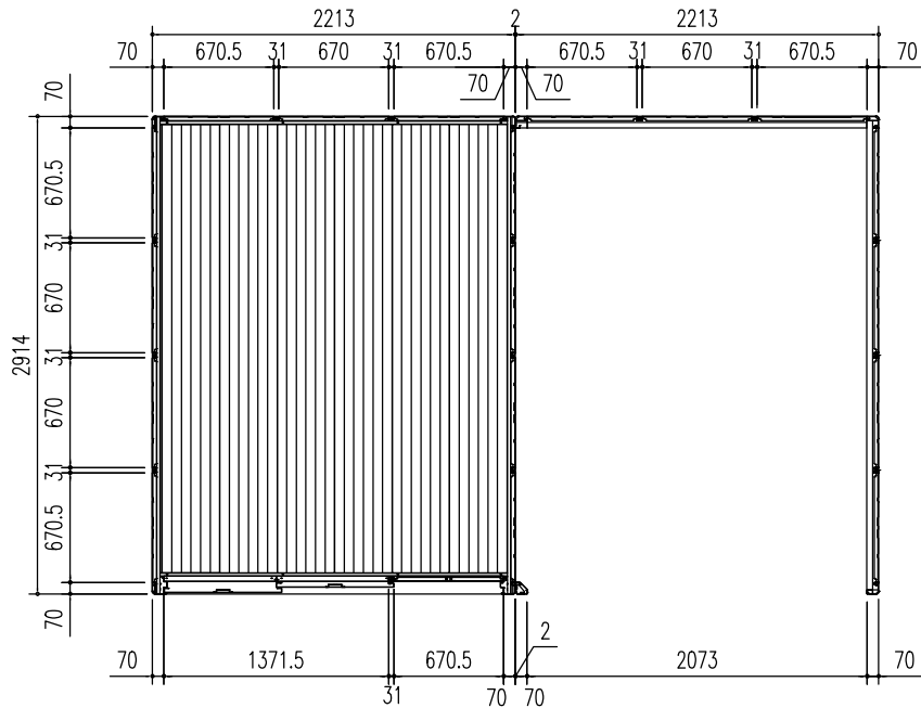
平面図 (S=1/50)
