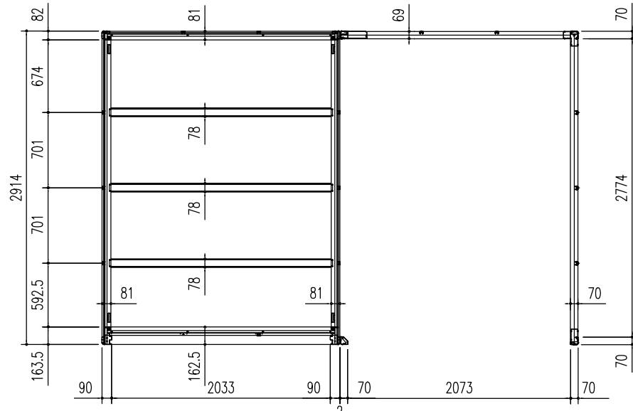
床伏図 (S = 1/50)
