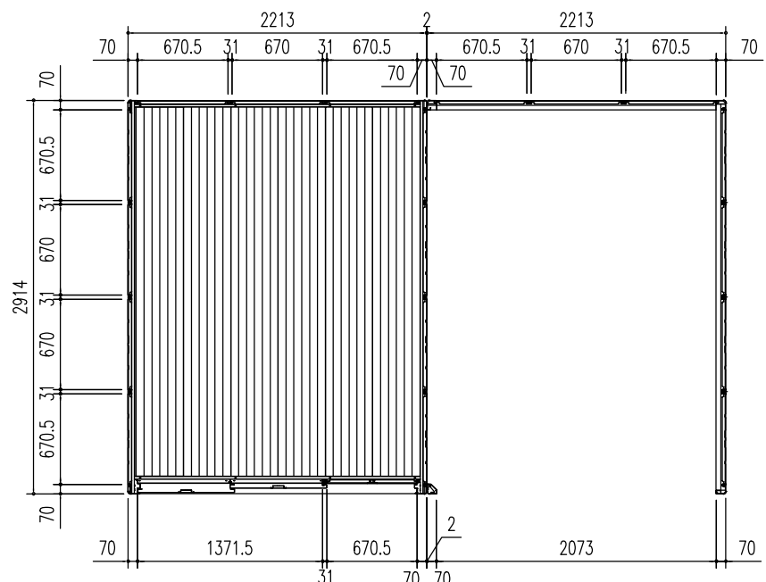
平面図 (S = 1/50)
