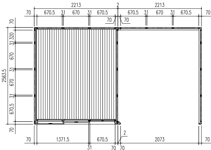
平面図 (S = 1/50)
