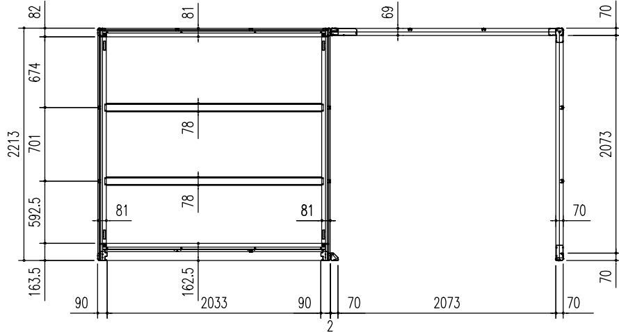
床 伏 図 (S = 1/50)
