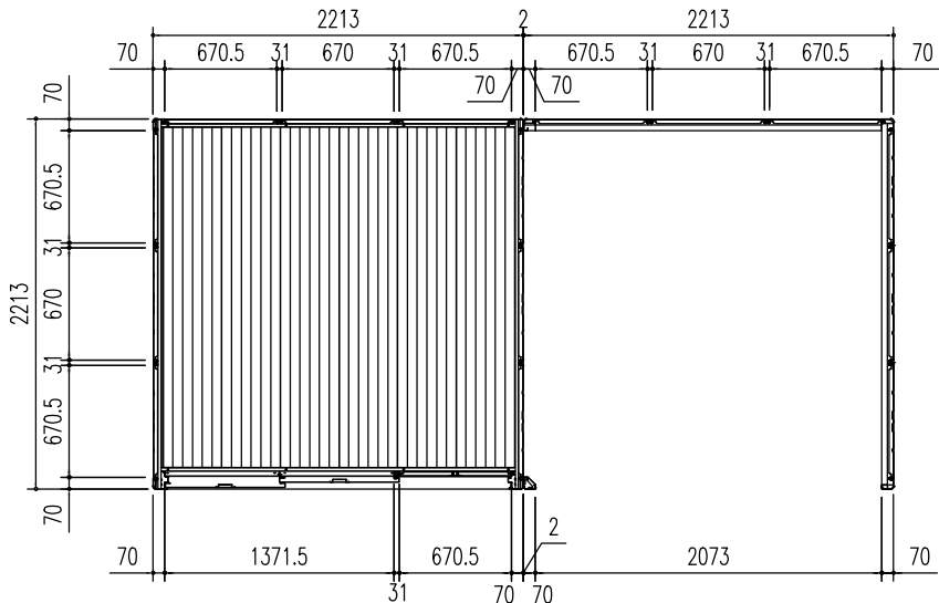
平面図 (S = 1/50)
