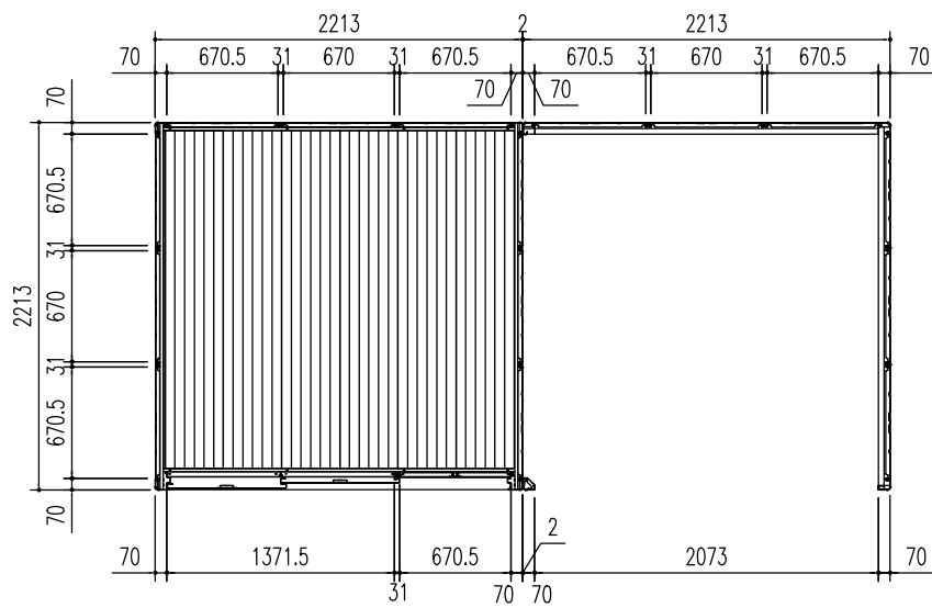
平面図 (S = 1/50)
