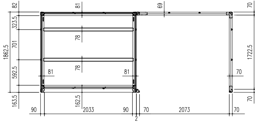
床 伏 図 (S = 1/50)
