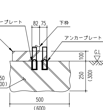
D ~ D' 断面 (外アンカー用)
