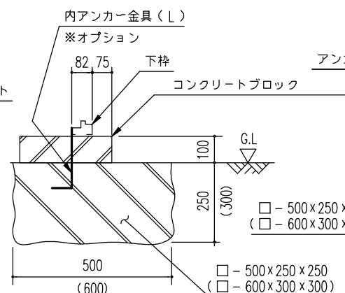
C ~ C' 断面 (内アンカー用)
