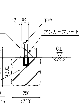
B ~ B' 断面 (外アンカー用)
