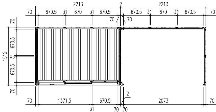
平 面 図 (S=1/50)
