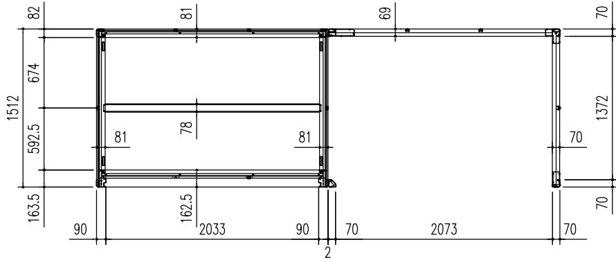
床 伏 図 (S=1/50)
