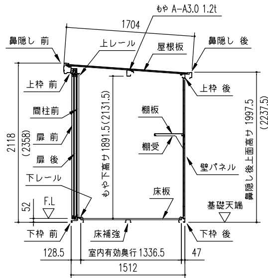
〔物置部〕矩計図 (S=1/50) ※( ) 内寸法は、Hタイプを示す。
