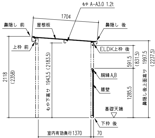
〔オープン部〕矩計図 (S=1/50) ※( ) 内寸法は、Hタイプを示す。
