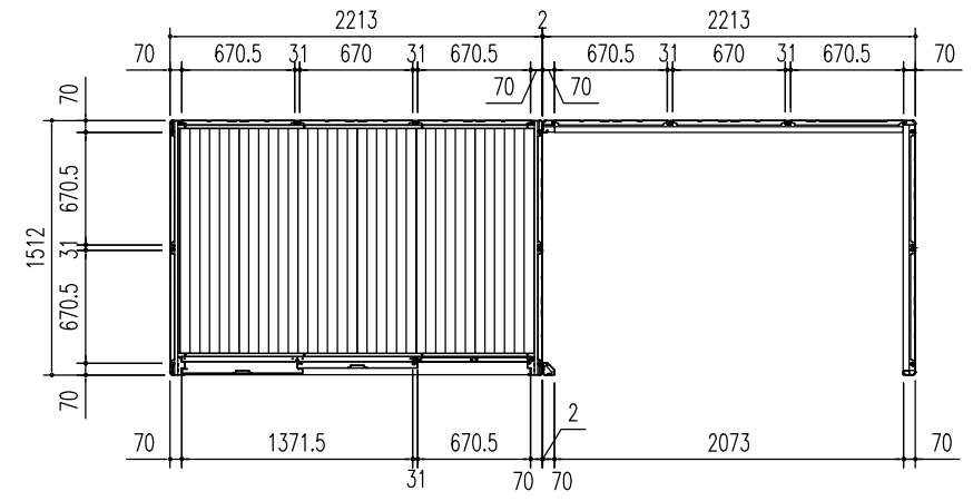
平 面 図 (S=1/50)
