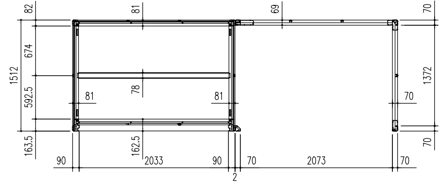
床 伏 図 (S=1/50)
