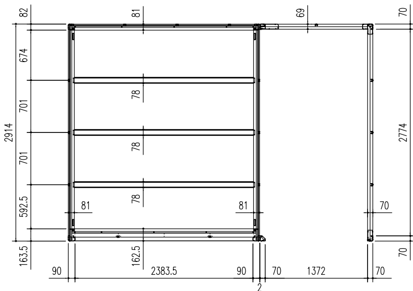
床伏図 (S=1/50)
