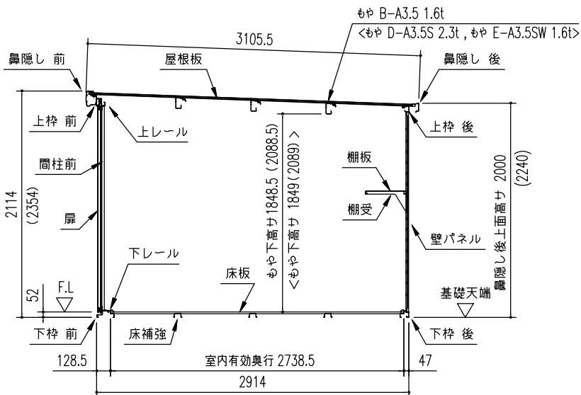
〔物置部〕矩計図 (S=1/50)
