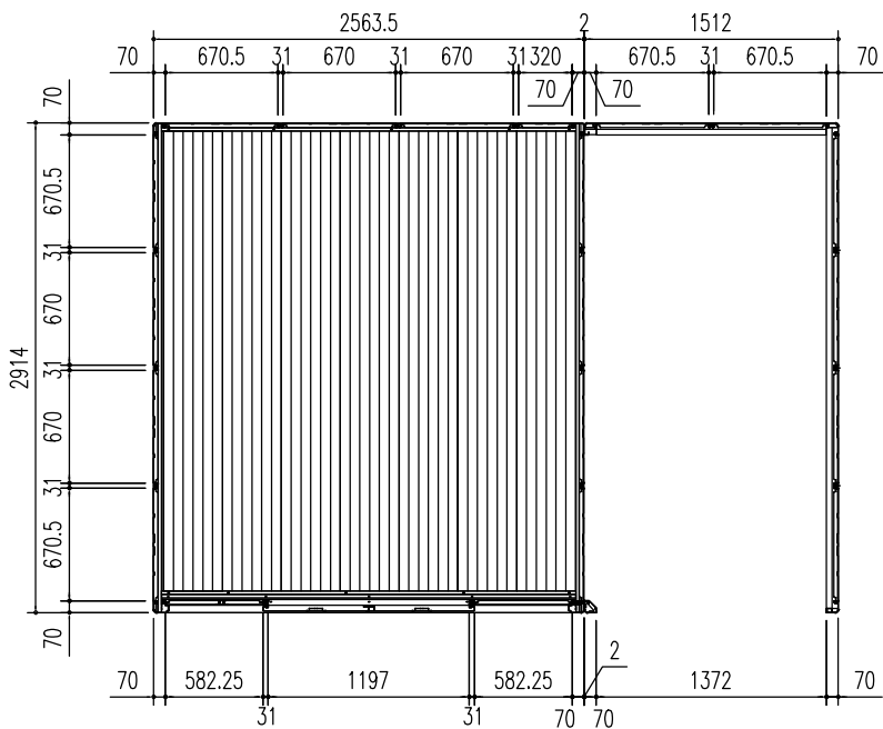
平面図 (S=1/50)
