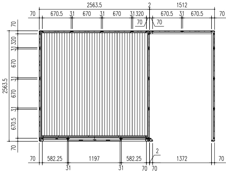
平面図 (S = 1/50)
