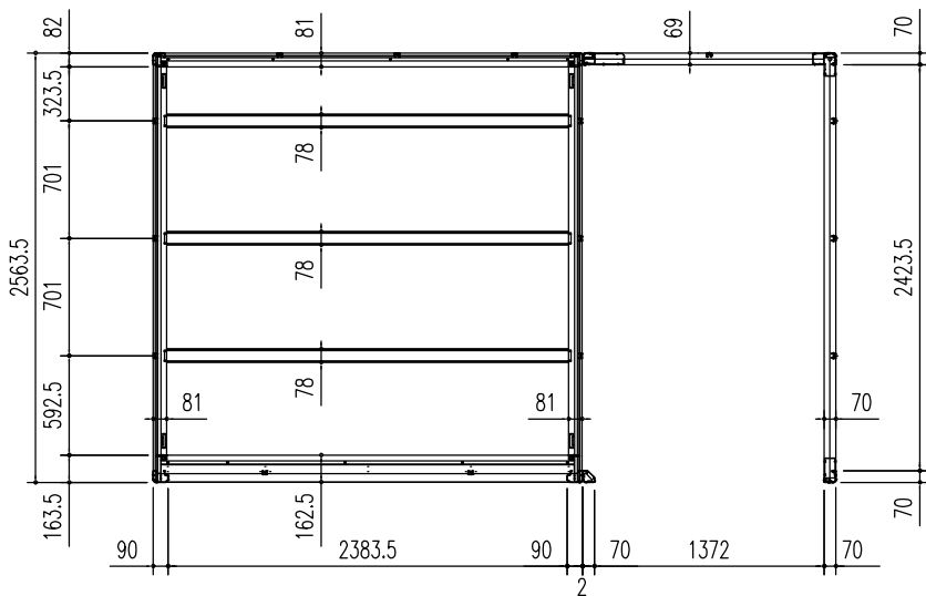
床伏図 (S = 1/50)
