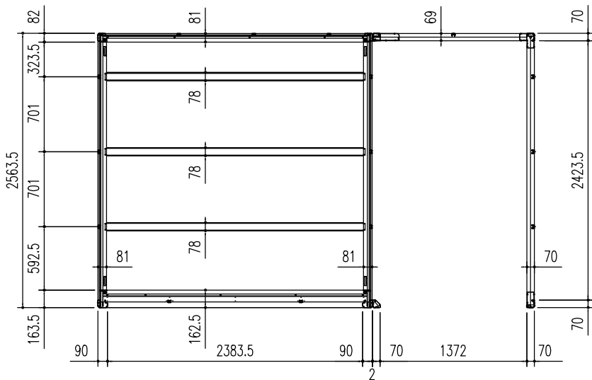
床伏図 (S=1/50)
