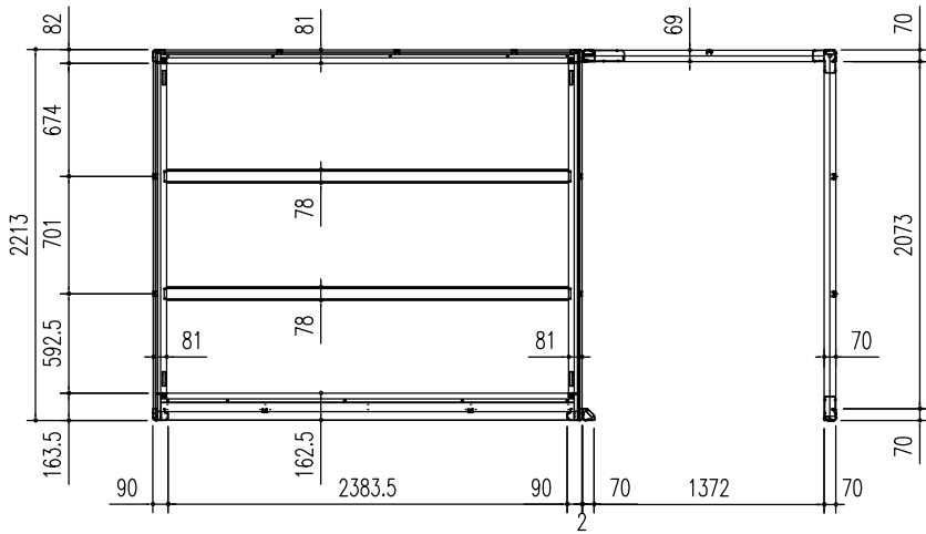
床伏図 (S = 1/50)
