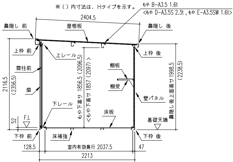
[物置部] 矩計図 (S = 1/50)
