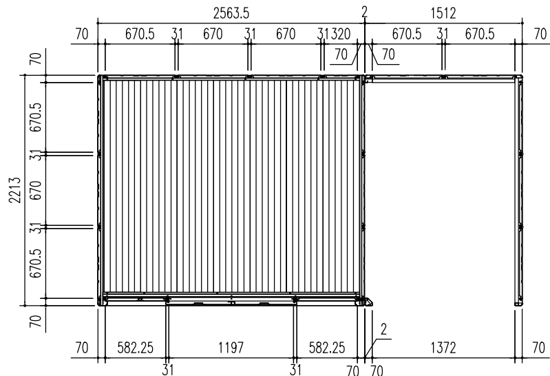
平面図 (S = 1/50)
