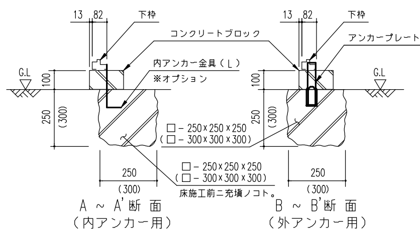
ブロック基礎断面図例 (S=1/20)
