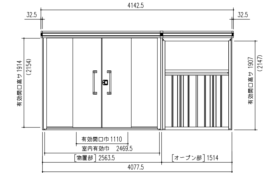
正面立面図 (S = 1/50)
