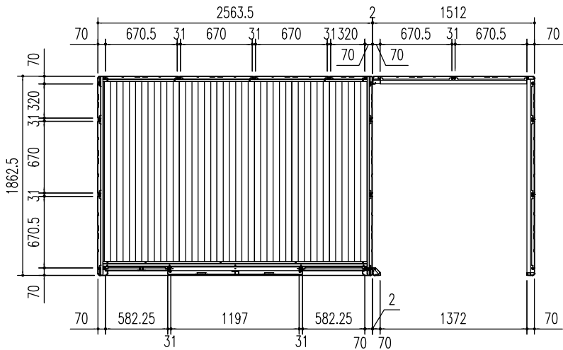
平面図 (S = 1/50)
