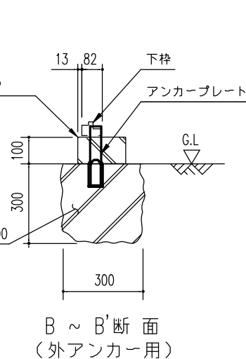
ブロック基礎断面図例 (S=1/20)
