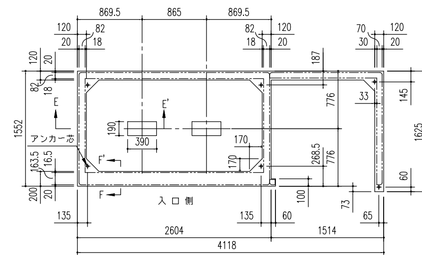
布基礎伏図 (S=1/50)
