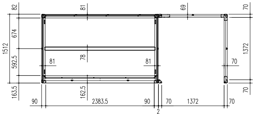
床伏図 (S=1/50)
