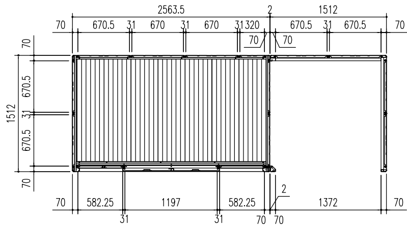
平面図 (S = 1/50)
