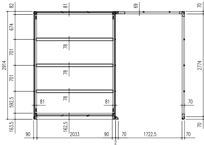
床伏図 (S = 1/50)
