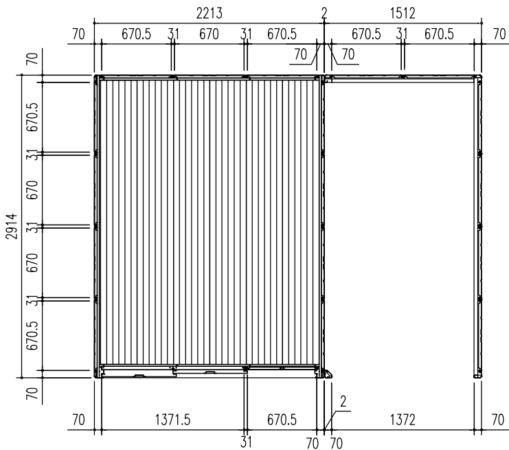
平面図 (S = 1/50)
