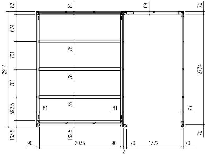
床 伏 図 (S = 1/50)
