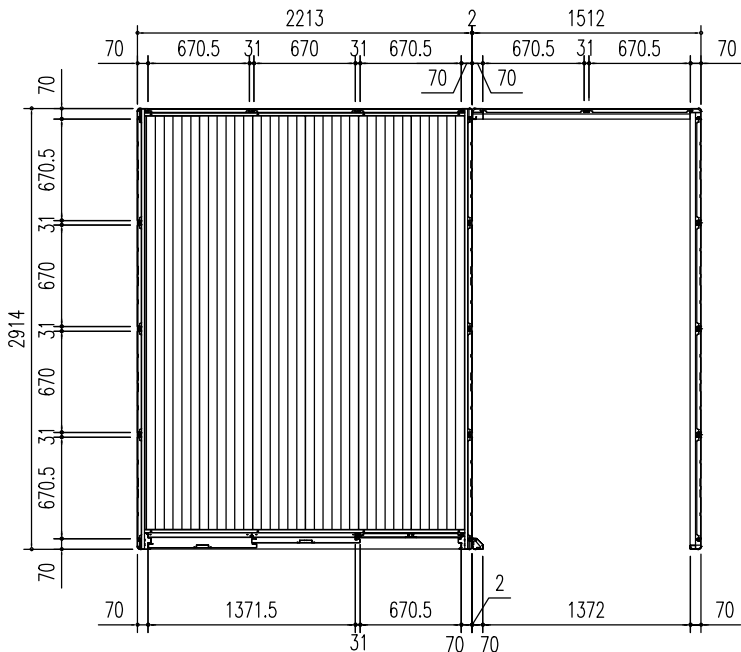
平面図 (S = 1/50)
